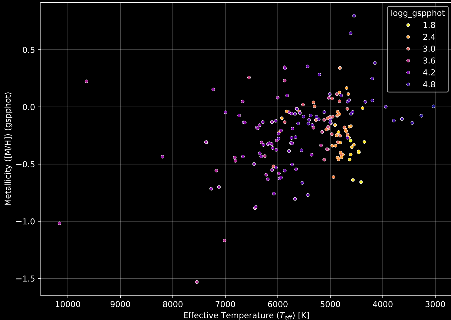
APOGEE DR17 Field: [CVZTILE_102+35_btx] Stellar Population Parameters (n= 184)
